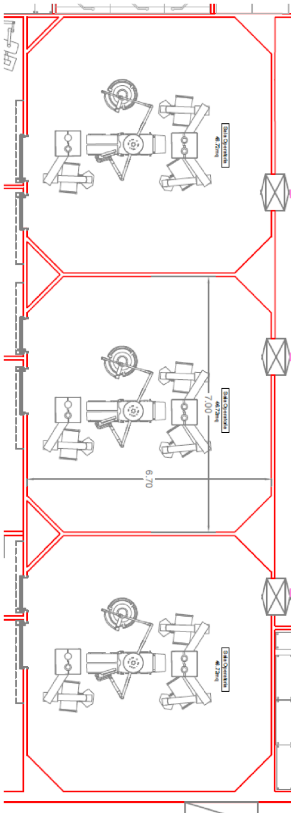
FIGURA 1: Layout Sale Operatorie prefabbricate da realizzare presso il P.O. Santobono
